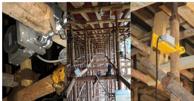
高支模监测
